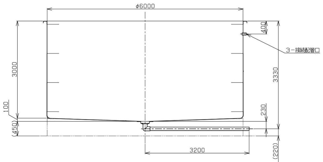
水槽組立図
